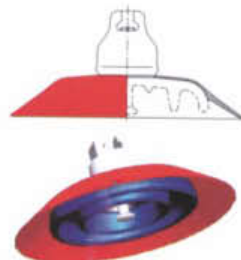
悬式瓷绝缘子增爬裙
