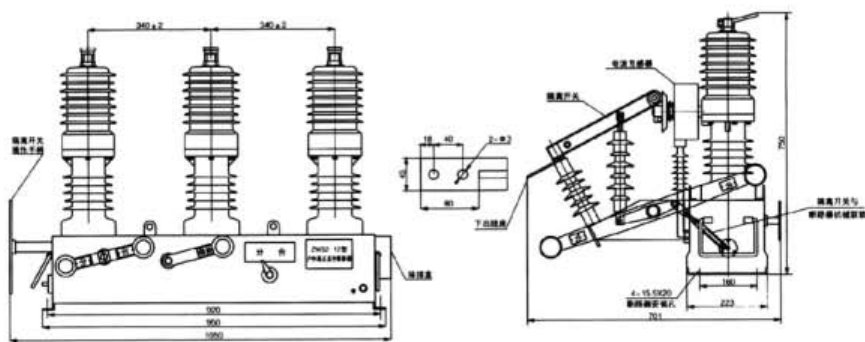
ZW32-12G型真空断路器结构及安装尺寸
