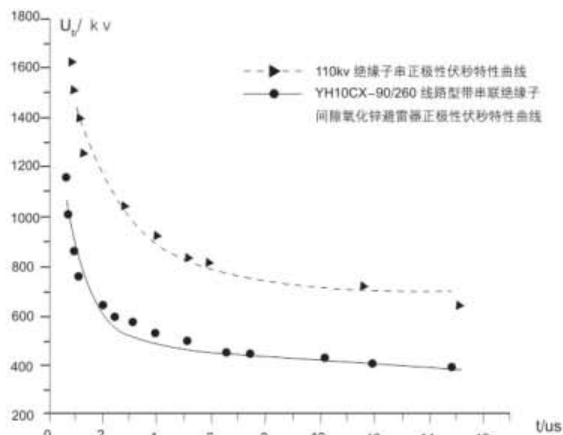
图 20 110kV 绝缘子串与绝缘子支撑间隙线路避雷器的伏秒特性配合曲线
