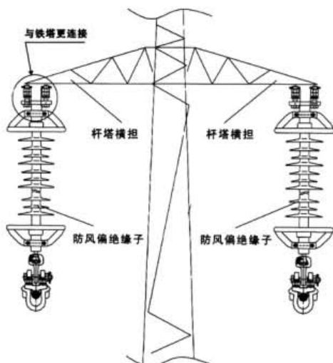
安装示意图 Installation Drawing
