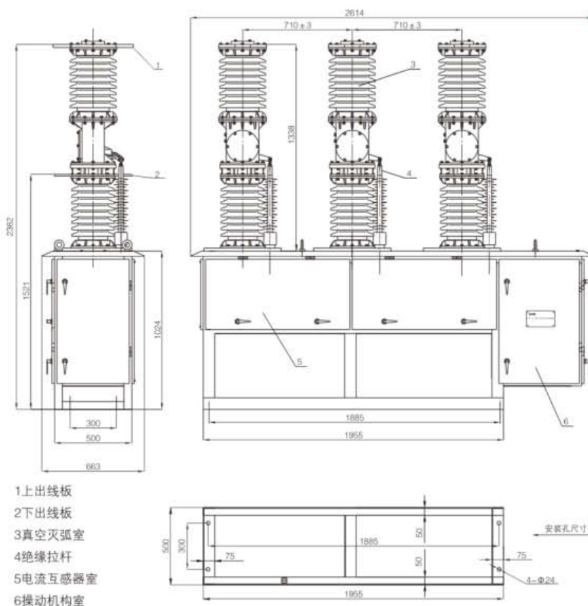
ZW7-40.5型(水平式内置互感器)户外高压真空断路器结构示意图三
