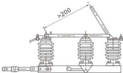
图三 GW1-12G(D2)
