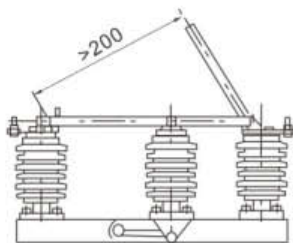
图一 GW1-12G
