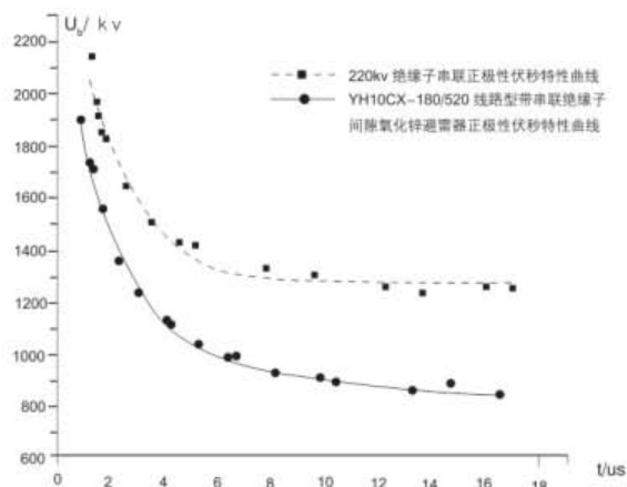
图 21 220kV 绝缘子串与绝缘子支撑间隙线路避雷器的伏秒特性配合曲线
