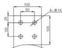
断路器上、下进出线板尺寸
