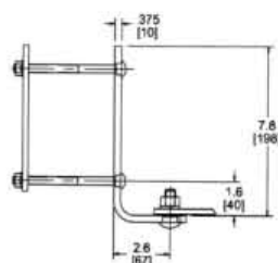
NEMA B bracket 安装支架B型
