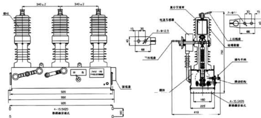
ZW32-12型真空断路器内部结构及安装尺寸
