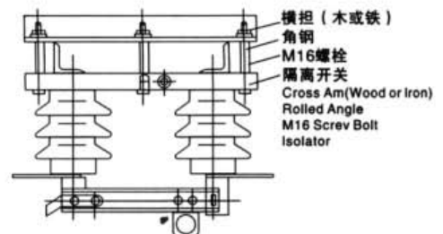
图3 隔离开关的安装
