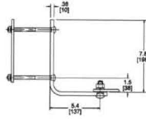
Extended bracket 加长型安装支架
