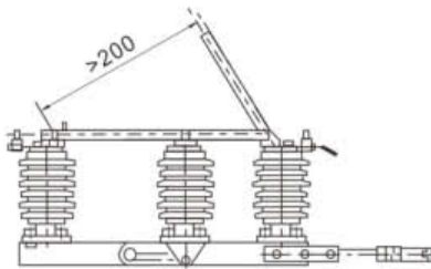
图二 GW1-12G(D1)
