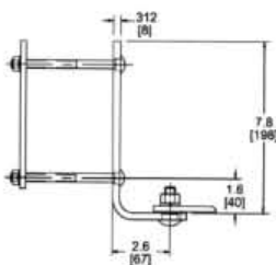
NEMA A bracket 安装支架A型
